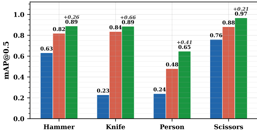
(a) Per-Class mAP@0.5 – v1 vs v2 vs v5 (Test Set)
